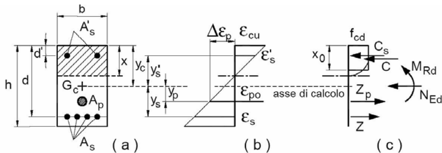
Fig. 4.1.4 – Sezione pressoinflessa
